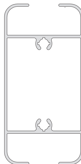
3050 / 67 Travesaño puerta vidrio simple 886 g/m 6 barras de 6.050 mm.
