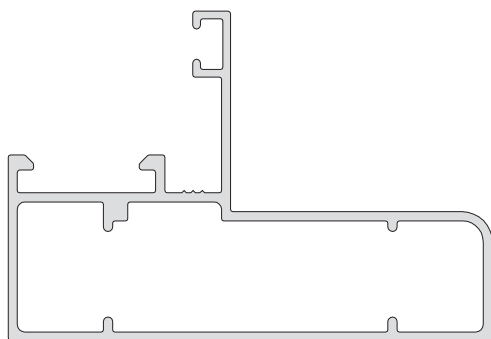
3050 / 60 Marco 64 mm. 721 g/m 4 barras de 6.050 mm.
