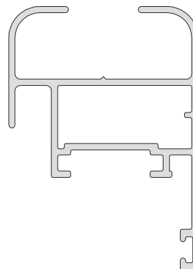
3050 / 62 Hoja ventana batiente vidrio simple 605 g/m 4 barras de 6.050 mm.
