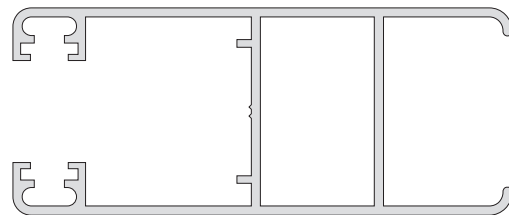
3050 / 425 Parante 707 g/m 8 barras 6.150
