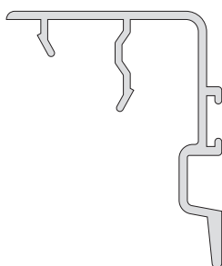
3050 / 262 Cierre 45° 316 g/m 15 barras de 6.150 mm.
