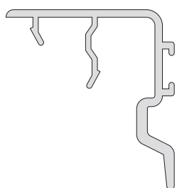
3050 / 172 Cierre 346 g/m 15 barras de 6.150 mm.
