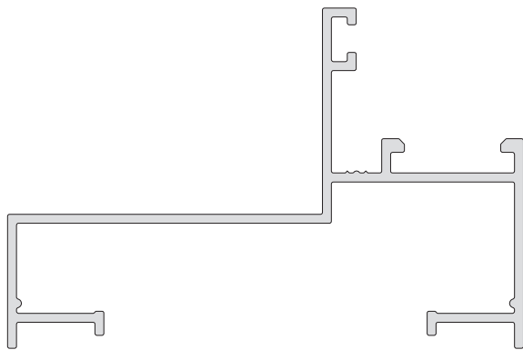
3050 / 176 Marco 75 715 g/m 4 barras 6.150
