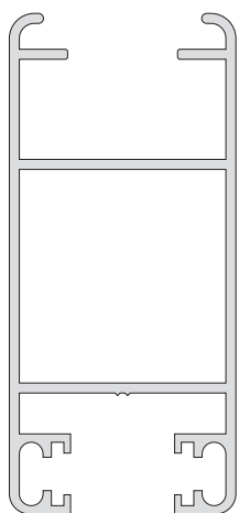
3050 / 53 Parante lateral corte 90° 699 g/m 8 barras de 6.150 mm.
