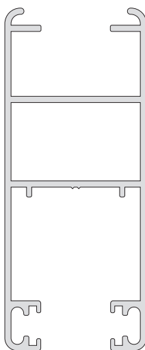
3050 / 261 Parante 45° 745 g/m 6 barras de 6.150 mm.
