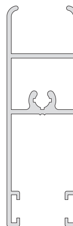
3050 / 52 Zócalo corte 90° 592 g/m 8 barras de 6.150 mm.
