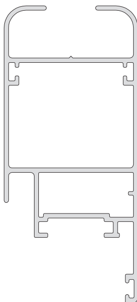
3050 / 66 Hoja puerta vidrio simple 945 g/m 4 barras de 6.050 mm.
