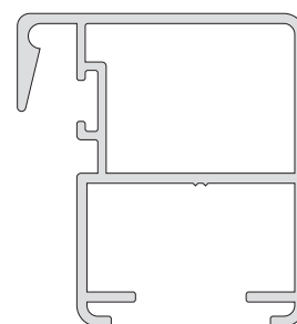
3050 / 54 Parante central corte 90° 532 g/m 10 barras de 6.150 mm.
