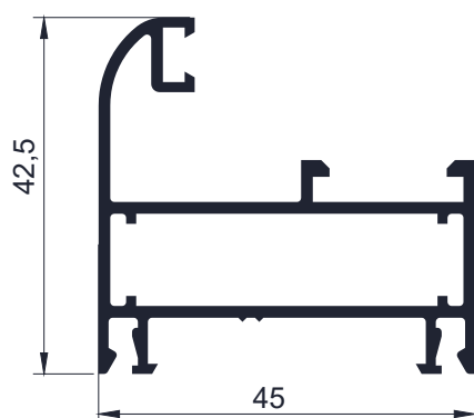
Código AW 6229 - Marco paño fijo curvo 0,735 Kg/m - Largo 6,2
