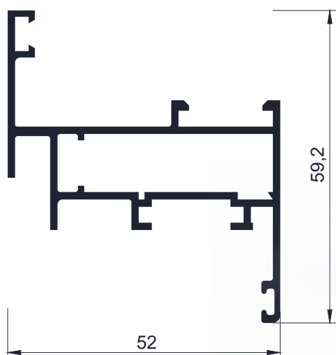
Código AW 6215 - hoja ventana de abrir doble contacto/banderola - 0,845 Kg/m Largo 6,2 - Tiras por paquete 2 und.
