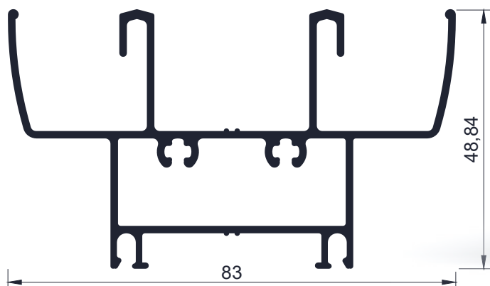
Código AW 6200 - Umbral y dintel de marco ventana y puerta corrediza - 1,255 Kg/m Largo 6,2 - Tiras por paquete 2 und.
