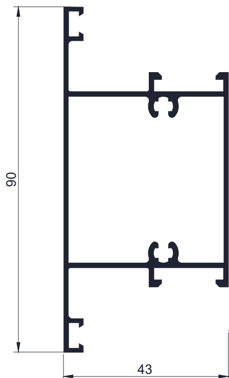
Código AW F52- Travesaño de puerta de 50mm 1,080 Kg/m -Largo 6,2 - Tiras por paquete 2 und
