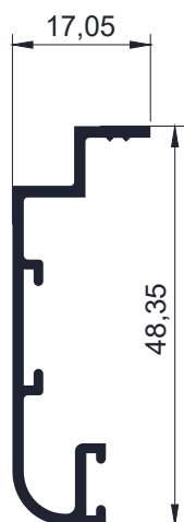
Código AW 4148 - Tapa pre marco - 0,338 Kg/m Largo 6,2 - Tiras por paquete 10 und
