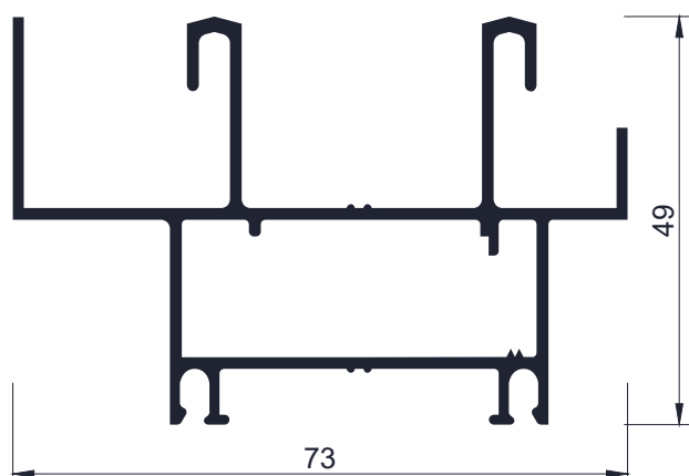
Código AW 906 - Marco perimetral corrediza 45° Recto - 1,10 Kg/m. Largo 6,2 - Tiras por paquete 2 und
