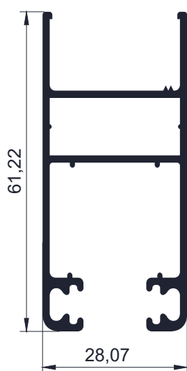
Código AW 6909 - Hoja DVH corrediza 45° - 0,820 Kg/m Largo 6,2 - Tiras por paquete 2 und
