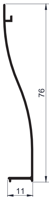
Código AW 826- Tablilla postigón curva 0,259Kg/m -Largo 6,2 - Tiras por paquete 10 und
