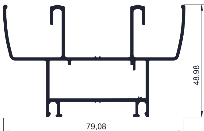
Código AW 6906 - Marco preperimetral corrediza 45° - 1,180 Kg/m Largo 6,2 - Tiras por paquete 2 und
