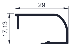
Código AW 6230 - Contravidrio curvo 29 mm. 0,210 Kg/m - Largo 6,2 - Tiras por paquete 10 und.
