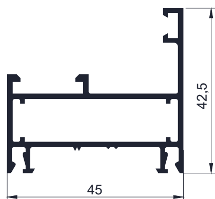
Código AW 6216 - Marco vent. abrir D.C. banderola/puerta rebatir ventiluz/PF recto 0.710Kg/m Largo 6.2 Tiras por paquete 2 und.
