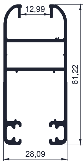
Código AW 6908 - Hoja de vidrio simple corrediza 45° - 0,875 Kg/m - Largo 6,2 - Tiras por paquete 2 und
