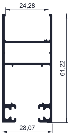
Código AW 909 - Hoja DVH corrediza 45° Recta 0,84 Kg/m. Largo 6,2 - Tiras por paquete 2 und
