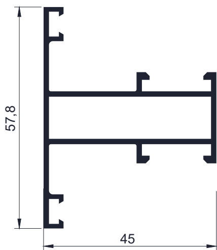
Código AW 6221 - Travesaño angosto paño fijo - 0,760 Kg/m Largo 6,2 - Tiras por paquete 3 und.
