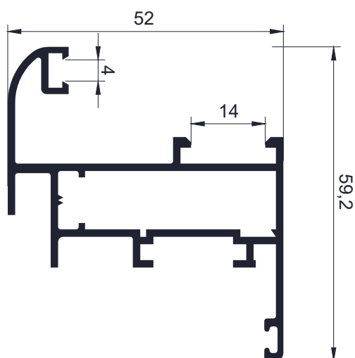
Código AW 6235 - Hoja curva ventana de abrir D.C./bandolera - 0,885 Kg/m - Largo 6,2 - Tiras por paquete 2 und.
