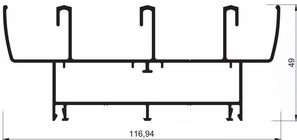
AW 6910 - Guia triple 45° - 1,621 Kg/m Largo 6,2- Tiras por paquete 2 und
