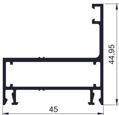
Código AW 6259 - Marco ventana proyectante 0,726 Kg/m - Largo 6.2 - Tiras por paquete 2 und.
