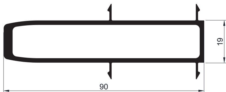
Código AW 6261 - Columna de acople reforzado 1,280 kg/m Largo 6,2 - Tiras por paquete 3
