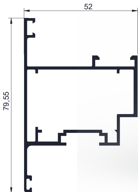
Código AW 6258 - Hoja de ventana proyectante recta 1,025 Kg/m - Largo 6.2 - Tiras por paquete 4 und.
