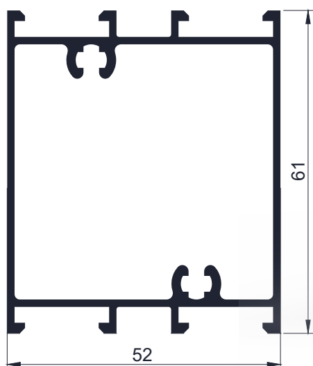
Código AW 6218 - Travesaño hoja puerta de rebatir - 1,150 Kg/m Largo 6,2 - Tiras por paquete 2 und.
