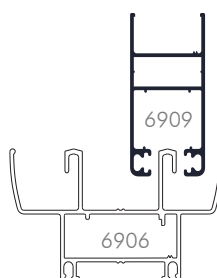
Código AW 6909 - Hoja DVH corrediza 45° - 0,820 Kg/m Largo 6,2 - Tiras por paquete 2 und
