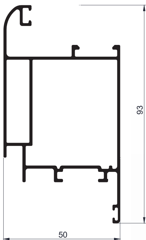
Código AW F53- Hoja de puerta de 50mm 1,222 Kg/m -Largo 6,2 - Tiras por paquete 2 und
