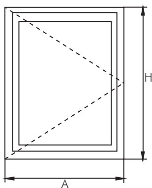
Ventana de abrir
