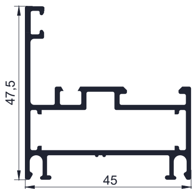
Código AW 6210 - Marco ventana de abrir con cámara compensadora - 0,765 Kg/m Largo 6,2 - Tiras por paquete 2 und.
