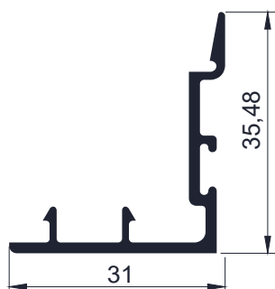
Código AW 907 - Complemento parante central corrediza 45° Recto 0,33 Kg/m - Largo 6,2 - Tiras por paquete 10 und
