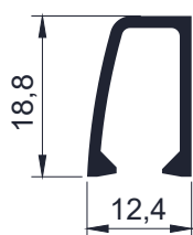
Código AW 6228 - Tope mosquitero ventana y puerta corrediza - 0,184 Kg/m Largo 6,2 - Tiras por paquete 10 und.
