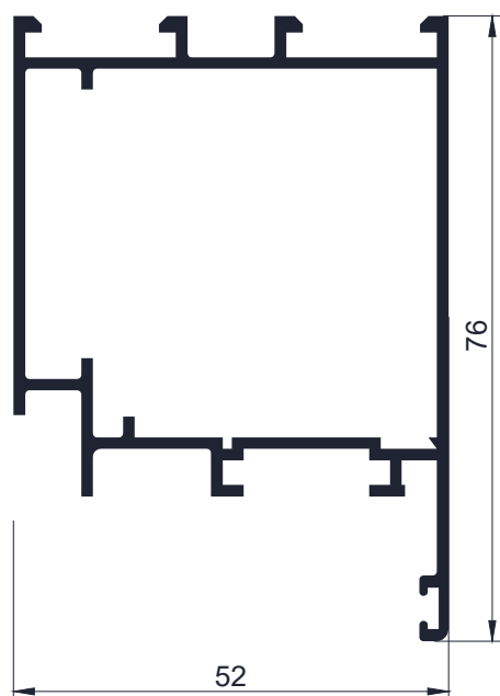
Código AW 6214 - Jambas y cabezal hoja puerta de rebatir - 1,080 Kg/m Largo 6,2 - Tiras por paquete 2 und.
