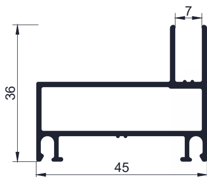
Código AW 6201 - Jambas de marco ventana y puerta corrediza - 0,655 Kg/m - Largo 6,2 Tiras por paquete 4 und.
