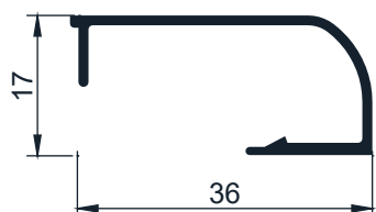
Código AW 6257 - Contravidrio curvo 36 mm 0,225 Kg/m - Largo 6,2 - Tiras por paquete 10 und.
