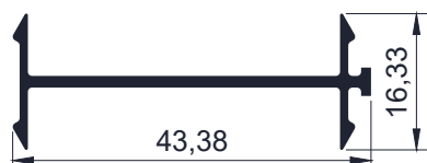
Código AW 6213 - Perfil de acople 0,255 Kg/m - Largo 6,2 - Tiras por paquete 10 und.
