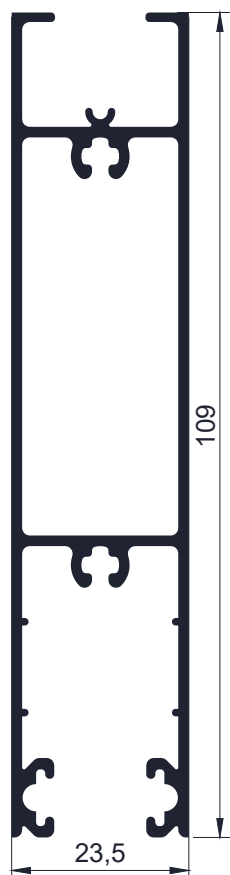
Código AW 6209 - Zócalo y cabezal de hoja para vidrio simple ventana y puerta corrediza - 1,260 Kg/m Largo 6,2 - Tiras por paquete 2 und.
