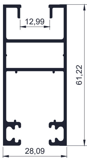
Código AW 908 - Hoja de vidrio simple corrediza 45°Recta 0,89 Kg/m - Largo 6,2 - Tiras por paquete 2 und
