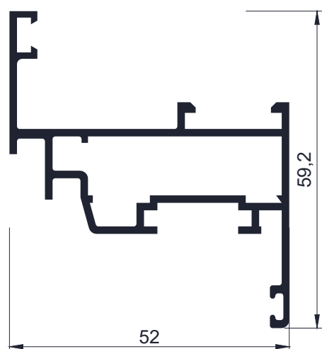
Código AW 6211 - Hoja ventana de abrir con cámara compensadora - 0,848 Kg/m Largo 6,2 - Tiras por paquete 2 und.
