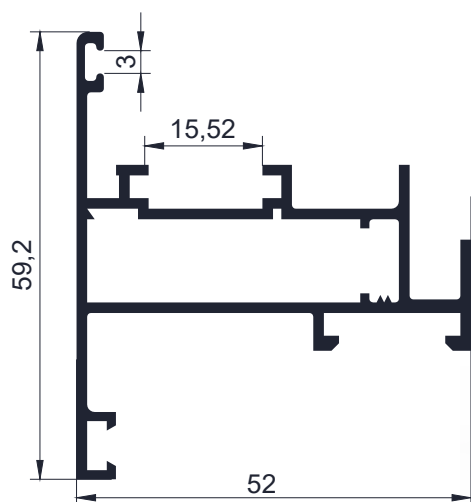
Código AW 6227 - Hoja ventiluz - 0,840 Kg/m Largo 6,2 - Tiras por paquete 2 und.
