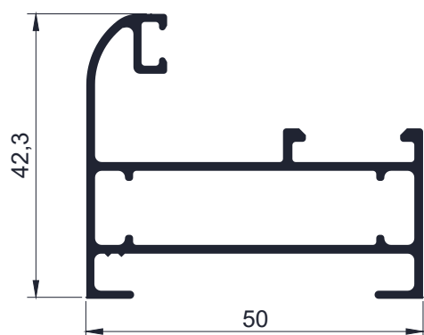
Código AW F50- Marco de puerta de 50mm 0,741 Kg/m -Largo 6,2 - Tiras por paquete 2 und
