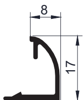
Código AW 6233- Contravidrio curvo 8mm 0,135 Kg/m - Largo 6,2 - Tiras por paquete 10 und.
