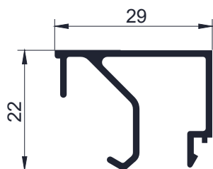
Código AW 6217 - Contravidrio 29 mm 0,291 Kg/m - Largo 6,2 - Tiras por paquete 10 und.
