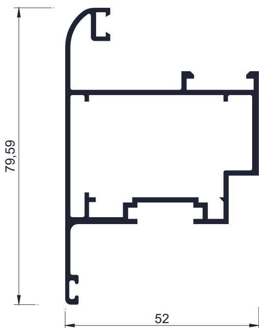
Código AW 6260 Hoja ventana proyectante curva 1.090 Kg/m -Largo 6,2 - Tiras por paquete 4 und
