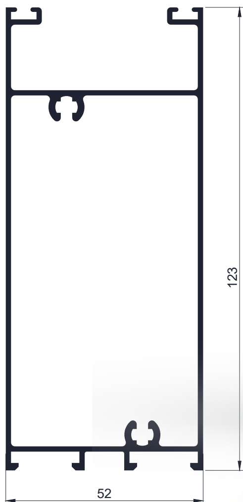
Código AW 6219 - Zócalo hoja puerta de rebatir- 1,645 Kg/m Largo 6,2 - Tiras por paquete 2 und.
