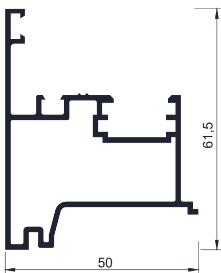
Código AW 6223 - Encuentro central ventana de abrir 2 hojas c/cámara compensadora - 0,915 Kg/m Largo 6,2 - Tiras por paquete 2 und.
