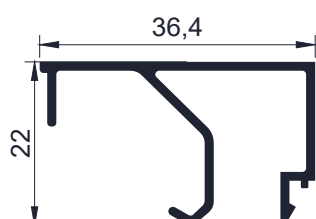
Código AW 6212 - Contravidrio 36 mm. 0,313 Kg/m - Largo 6,2 - Tiras por paquete 10 und.
