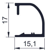
Código AW 6231 - Contravidrio curvo 15 mm. 0,158 Kg/m - Largo 6,2 - Tiras por paquete 10 und.
