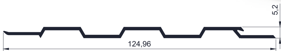
Código AW 782 - Tablilla revestimiento doble faz- 0,564 kg/m Largo 6,2 - Tiras por paquete 4
