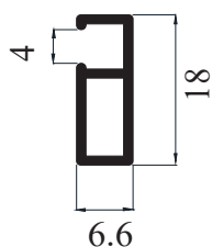
Código AW 6111- Mosquitero fijo 0,121 Kg/m -Largo 6,2 - Tiras por paquete 10 und
