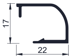
Código AW 6232 - Contravidrio curvo 22 mm 0,179 Kg/m - Largo 6,2 - Tiras por paquete 10 und.
