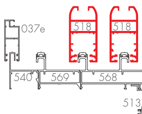
Código AW 518 - Hoja a 45° corrediza VS 1.57 Kg/m - Largo 6,2
