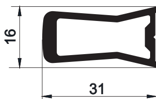
Código AW 567- Refuerzo Mosquitero 0.470 Kg/m - Largo 6,2
