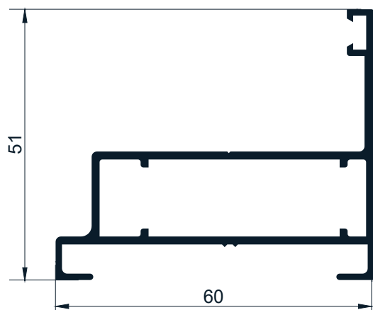
Código AW 526- Marco ventana desplazable 0,834 Kg/m - Largo 6,2
