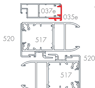
Código AW 035e - Tapa hoja Mosquitero 0.166 Kg/m - Largo 6,2
