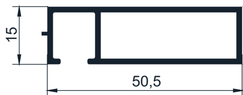
Código AW 515 Premarco 0,52 Kg/m - Largo 6,2
