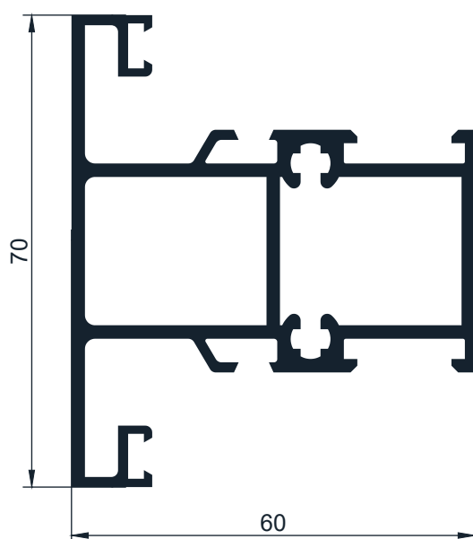
Código AW 522- Travesaño paño fijo 1,79 Kg/m - Largo 6,2
