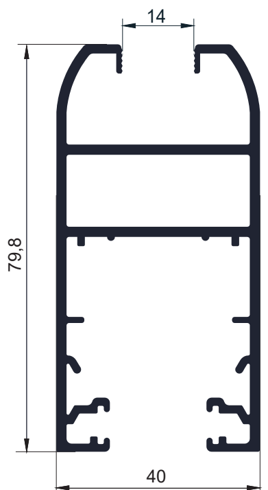
Código AW 518 - Hoja a 45° corrediza VS 1.57 Kg/m - Largo 6,2
