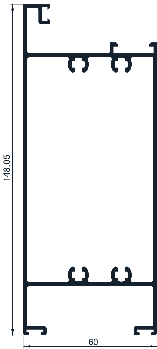
Código AW 543- Zócalo Puerta de Rebatir 2,319 Kg/m - Largo 6,2
