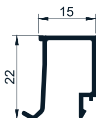
Código AW 6226- Contravidrio recto de 22mm, corte a 90° 0,211 Kg/m - Largo 6,2
