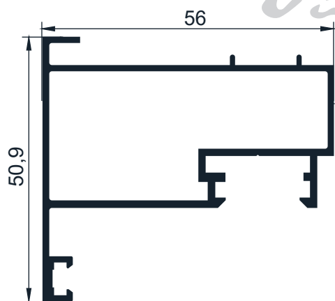
Código AW 529- Acople Puerta y Ventana de abrir de dos hojas 0,818Kg/m - Largo 6,2
