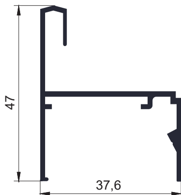
Código AW 540 - Guía de mosquitero (acoplable) 0,479 Kg/m - Largo 6,2 -
