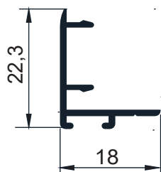
Código AW 035e - Tapa hoja Mosquitero 0.166 Kg/m - Largo 6,2
