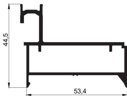
Código AW 569 - Marco corrediza una guía (acoplable) 0.888Kg/m - Largo 6,2 -
