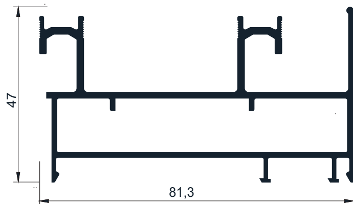
Código AW 568 - Marco dos guias corrediza a 45° 1,465 Kg/m - Largo 6,2 -
