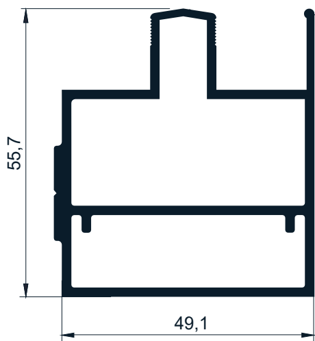
Código AW 555- Acople a 90° recto y guía simple para corredizas 1 hoja armado a 45° 1.553Kg/m - Largo 6,2
