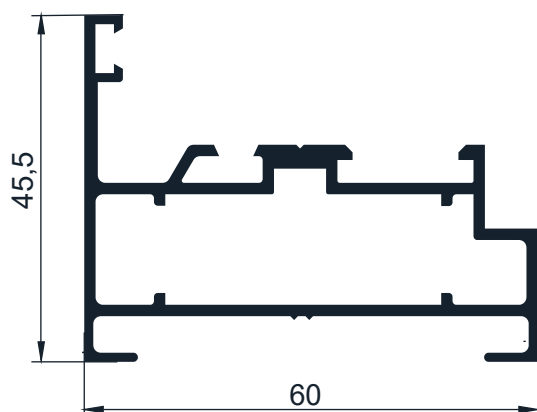
Código AW 523- Marco coplanar ventana de rebatir/oscilobatiente 0,995Kg/m - Largo 6,2
