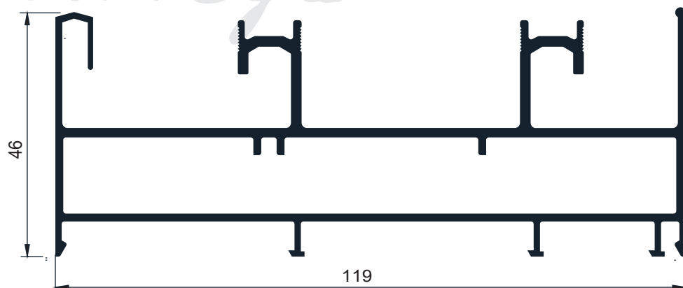
Código AW 570 - Marco coplanar de 3 guias (2 guias hoja + guía de mosquitero) 1,947 Kg/m - Largo 6,2 -
