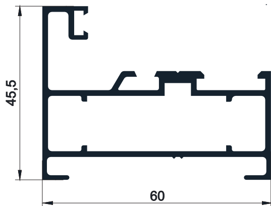
Código AW 524- Marco paño fijo y rebatir 1,034 Kg/m - Largo 6,2
