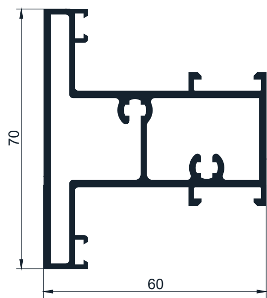
Código AW 530- Travesaño Puerta de Rebatir 1,715 Kg/m - Largo 6,2
