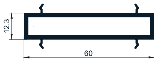
Código AW 536- Acople reforzado 0,791 Kg/m - Largo 6,2
