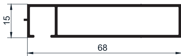
Código AW 564 Premarco 68mm. 0,564 Kg/m - Largo 6,2
