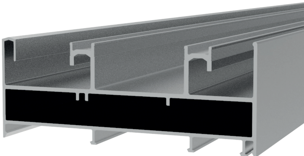
Código AW 570 - Marco coplanar de 3 guias (2 guias hoja + guía de mosquitero) 1,947 Kg/m - Largo 6,2 -
