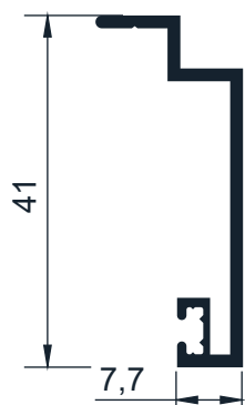
Código AW 514 Tapajuntas Recto 0,28Kg/m - Largo 6,2
