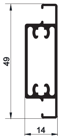
Código AW 566- Travesaño Mosquitero. Peso 0.486 Kg/m - Largo 6,2m
