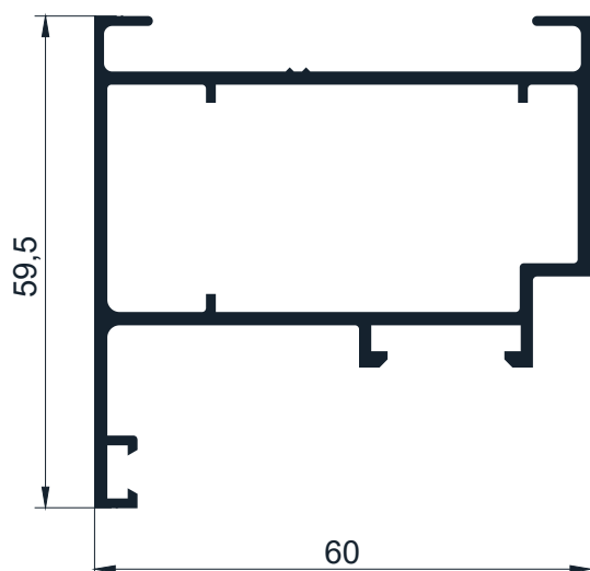
Código AW 527- Marco Puerta de Rebatir 1,140 Kg/m - Largo 6,2
