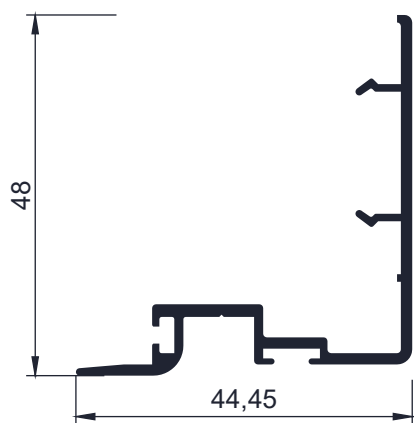
Código AW 520 - Encuentro recto hoja a 45° 0.48Kg/m - Largo 6,2
