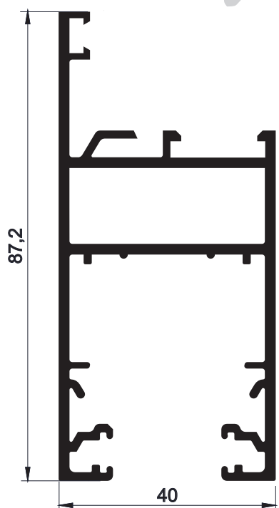
Código AW 558- Hoja recta corrediza, corte a 45° 1.577Kg/m - Largo 6,2
