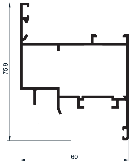
Código AW 557- Hoja de ventana de rebatir/oscilobatiente 1,192 Kg/m - Largo 6,2
