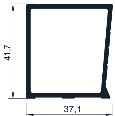
Código AW 533 Refuerzo 0,83 Kg/m - Largo 6,2
