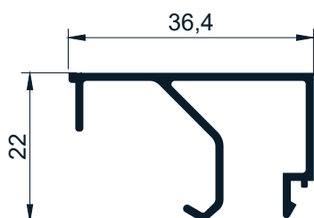
Código AW 6212- Contravidrio recto de 22mm, corte a 90° 0,315 Kg/m - Largo 6,2
