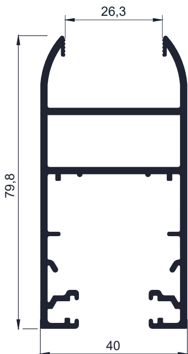
Código AW 517 - Hoja a 45° corrediza DVH 1.54 Kg/m - Largo 6,2
