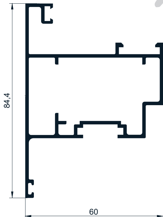
Código AW 525 Hoja ventana desplazable 1,296Kg/m - Largo 6,2
