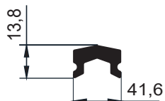
Código AW 565 - Guia Postiza 0,084 Kg/m - Largo 6,2 -
