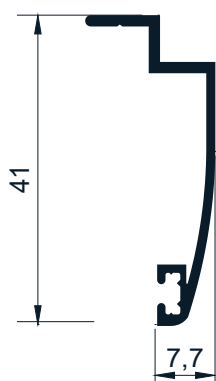
Código AW 513 Tapajuntas Curvo 0,24Kg/m - Largo 6,2
