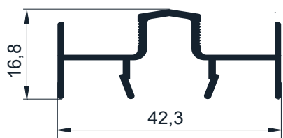
Código AW 407 Encuentro central 0,47 Kg/m - Largo 6,2
