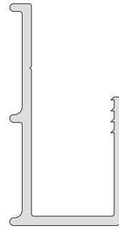
3060/14 437 g/m 12 barras de 6.050 mm.
